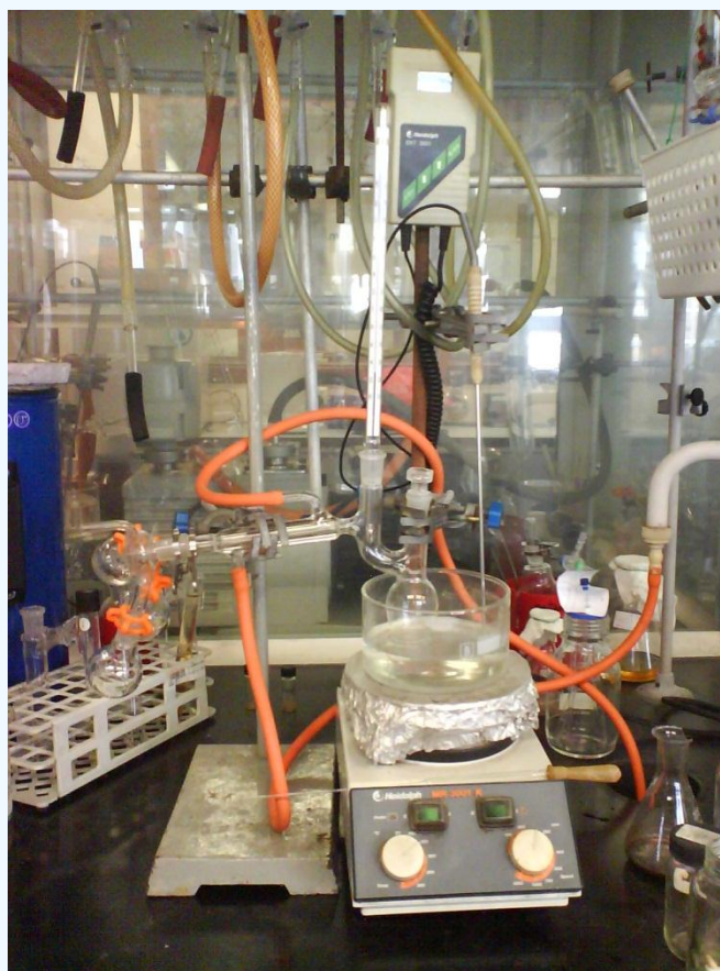
Вакуумная перегонка
