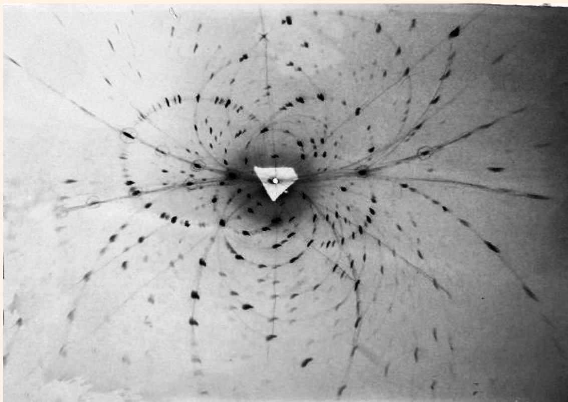
Рентгенограмма кристалла, полученная методом Лауэ (лауэграмма)
