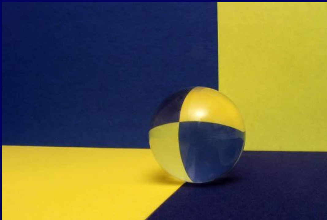
Преломление и отражение света в стеклянном шарике
