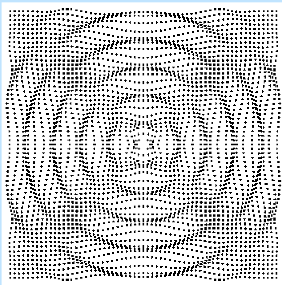
Визуализация звуковых волн
