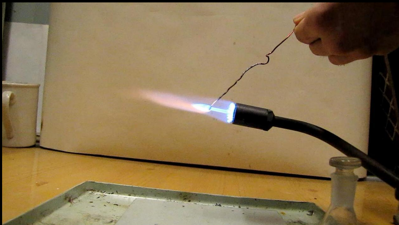
Проба Бейльштейна
