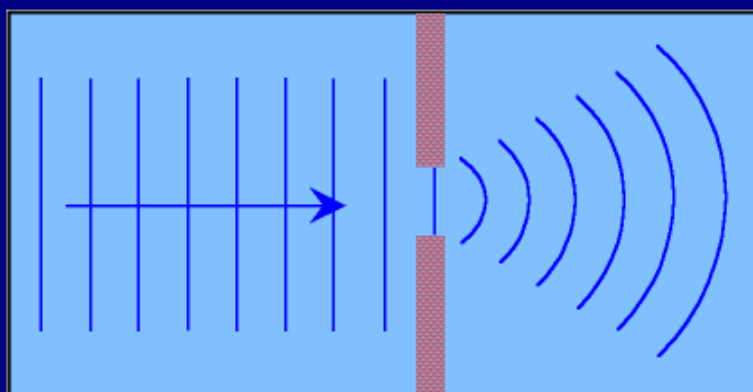
Дифракция волн на воде (фотография и схема)
