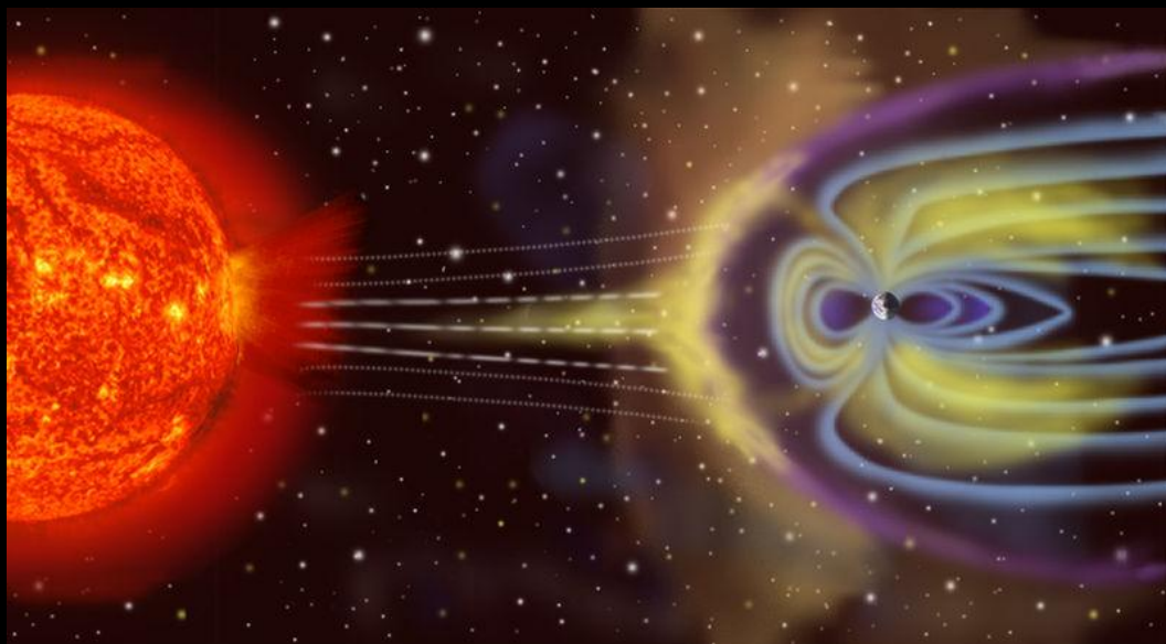
Взаимодействие магнитного поля Земли и солнечного ветра
