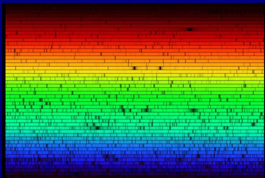
Солнечный спектр
