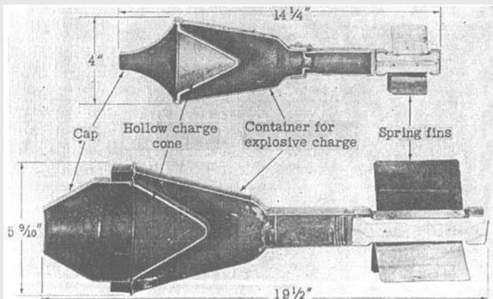
Фаустпатрон (панцерфауст) - ручной противотанковый гранатомет одноразового действия
