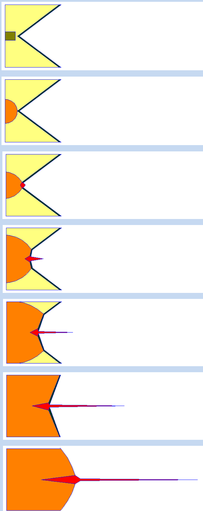
Формирование кумулятивной струи
