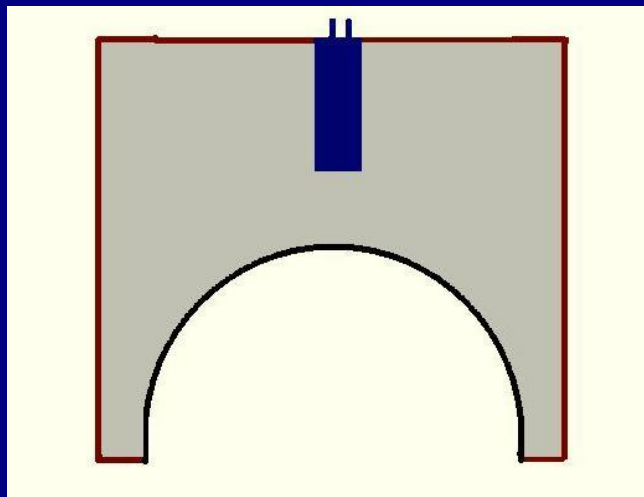
Схема кумулятивного заряда
