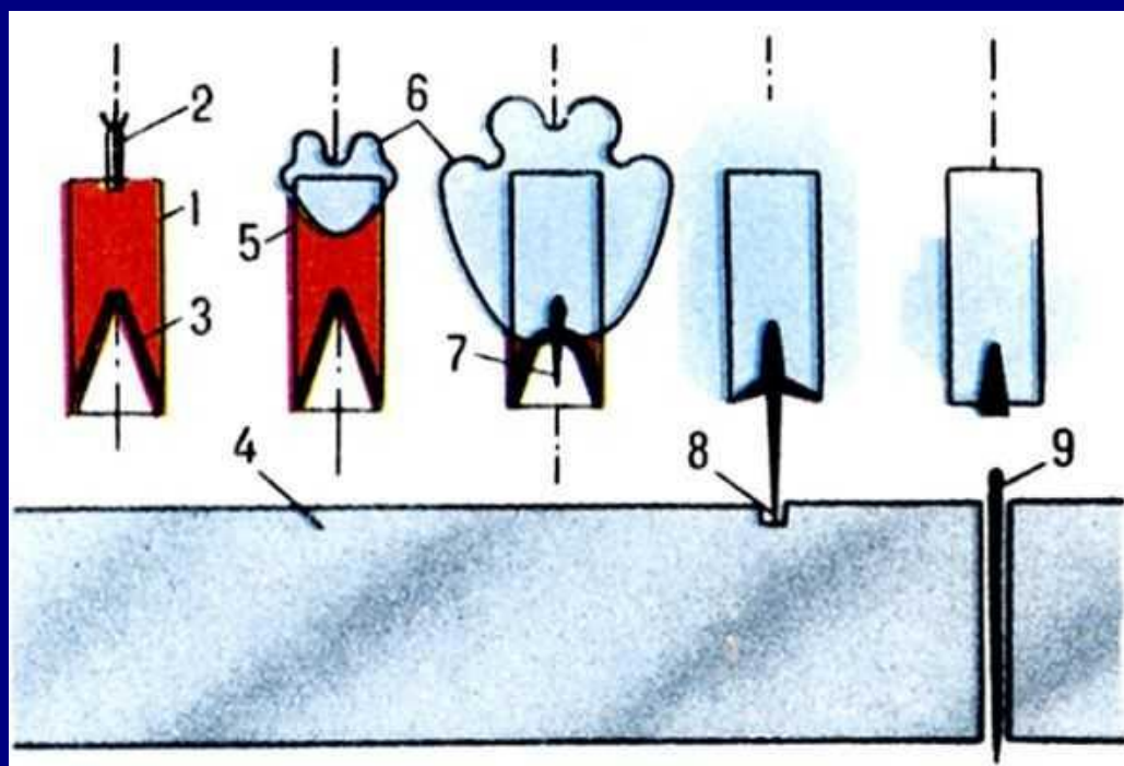
Взрыв кумулятивного заряда
