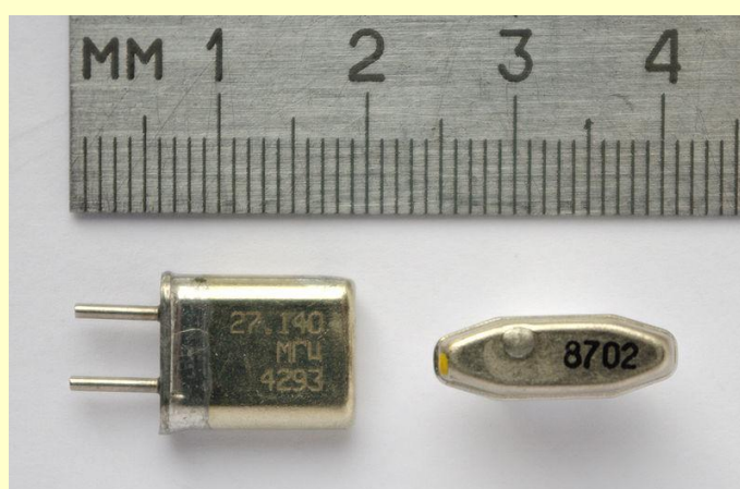
Кварцевые резонаторы
