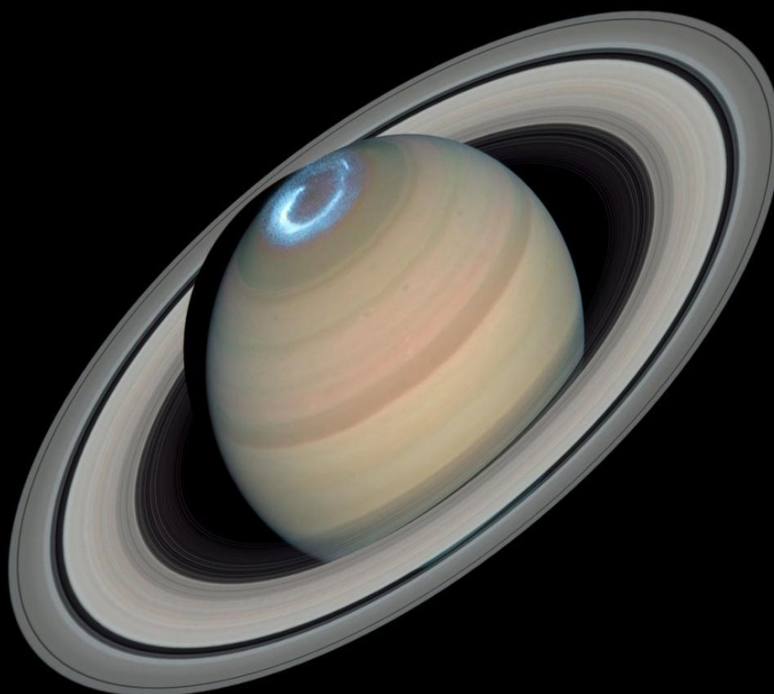
Полярное сияние на Сатурне
