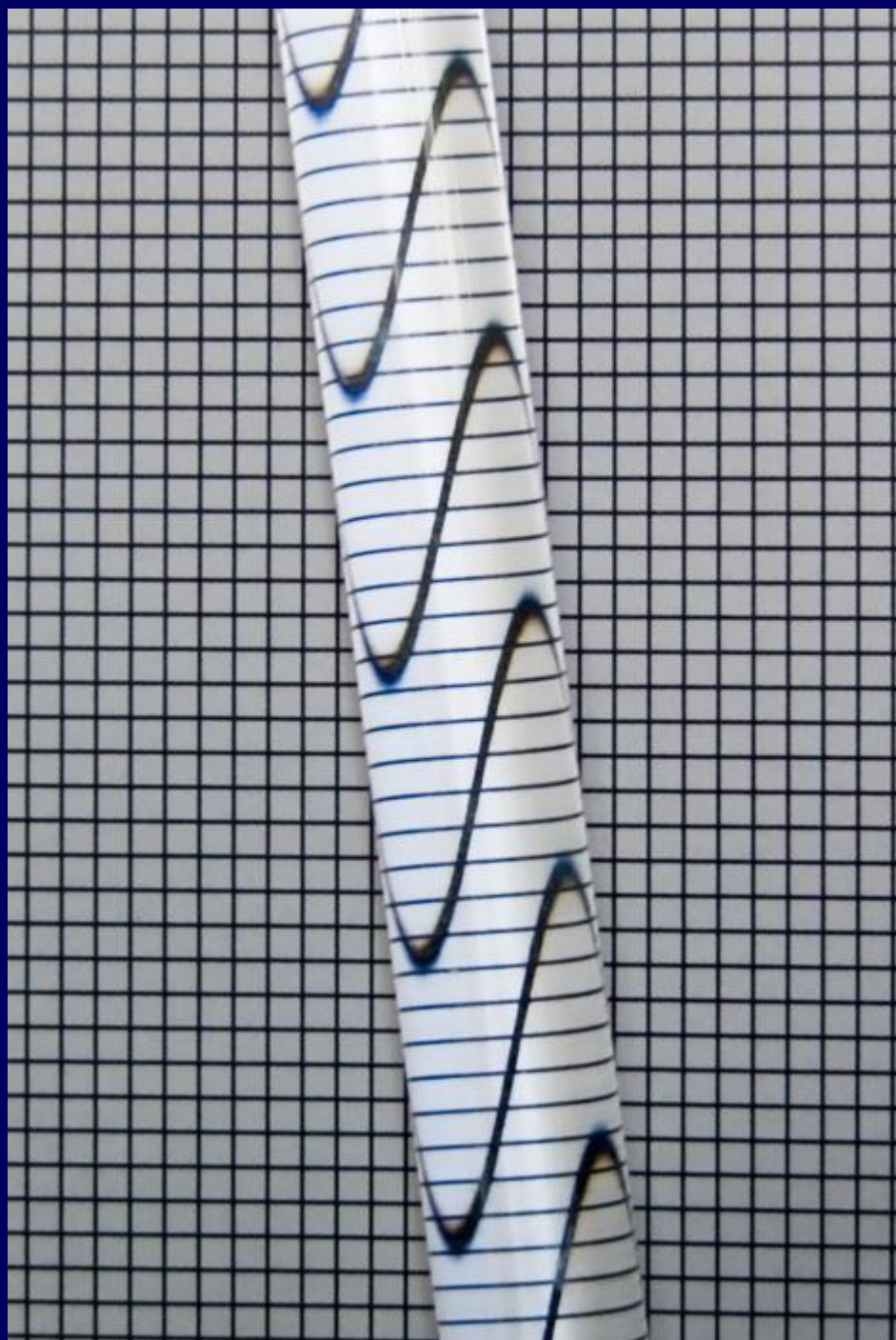
Преломление в стеклянном стержне
