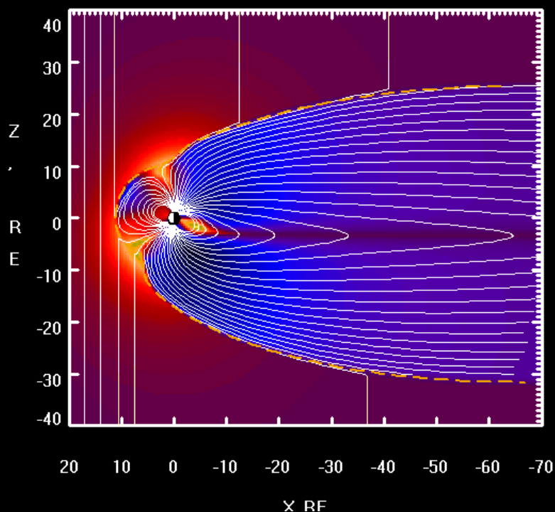
Взаимодействие магнитного поля Земли и солнечного ветра (по осям отложено расстояние в радиусах Земли)
