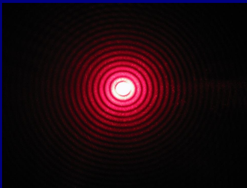
Дифракция света красного лазера
