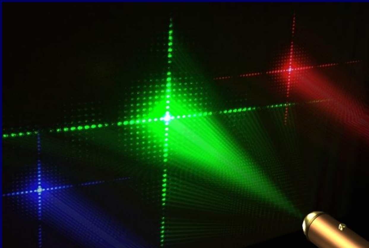
Дифракционная решетка и лазеры
