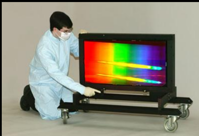
Дифракционная решетка (очень большая)
