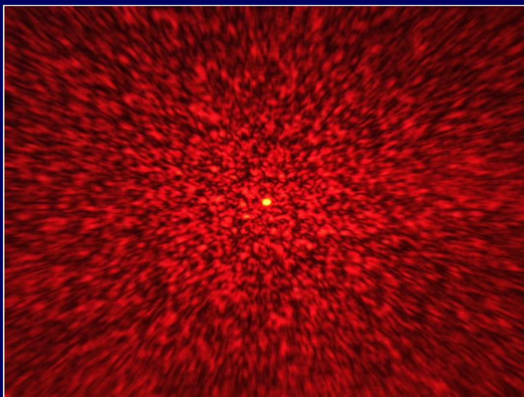
Спеклы (случайная интерференционная картина, которая образуется при взаимной интерференции когерентных волн, имеющих случайные сдвиги фаз и/или случайный набор интенсивностей)
