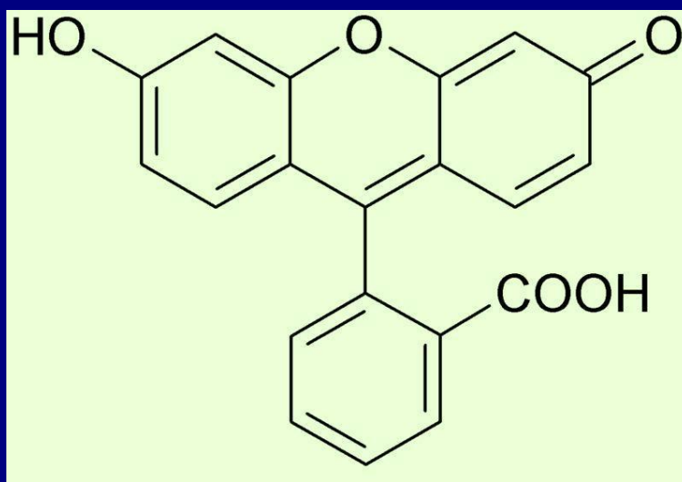
Флуоресцеин
