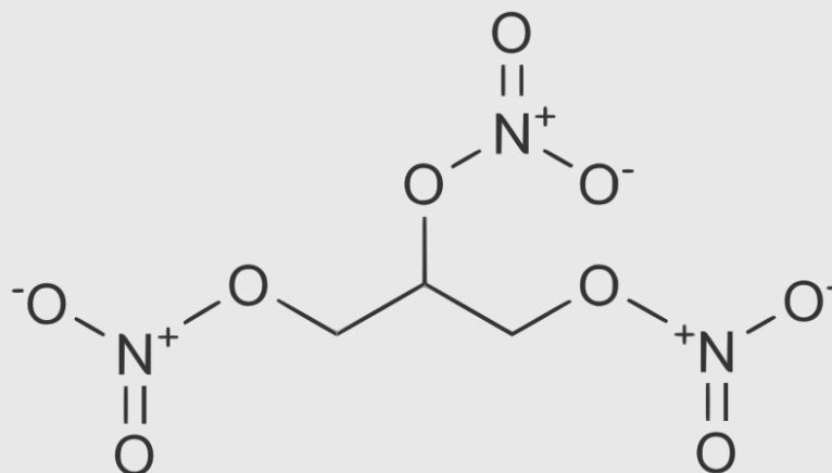
Нитроглицерин
