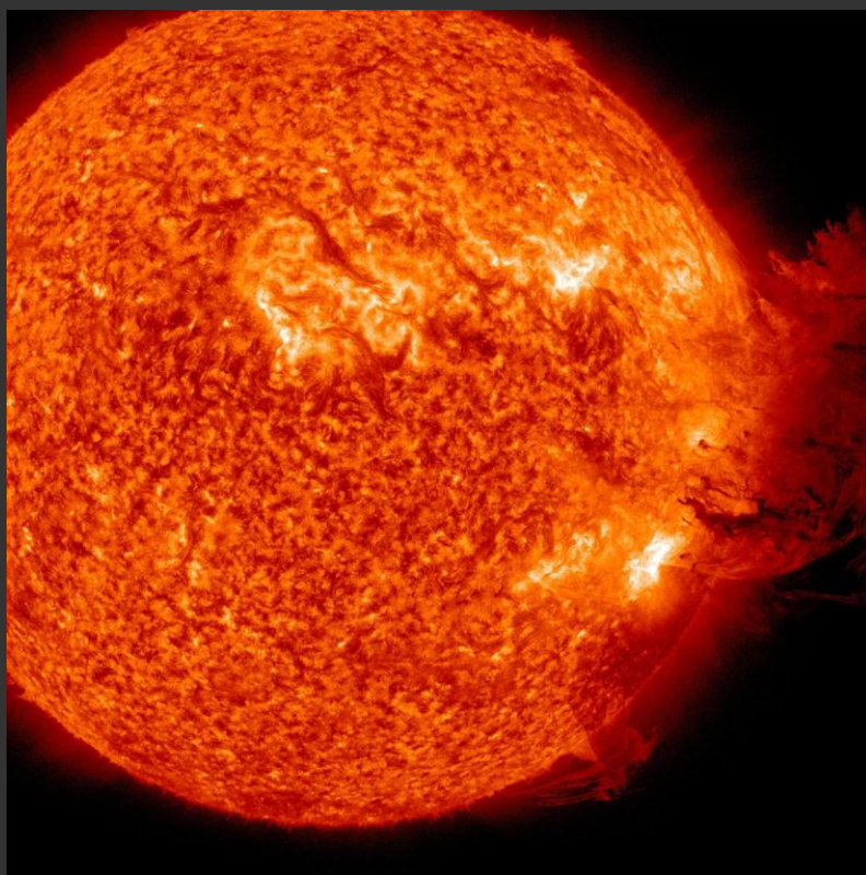
Вспышка на Солнце
