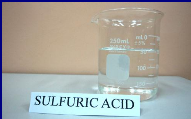
Серная кислота
